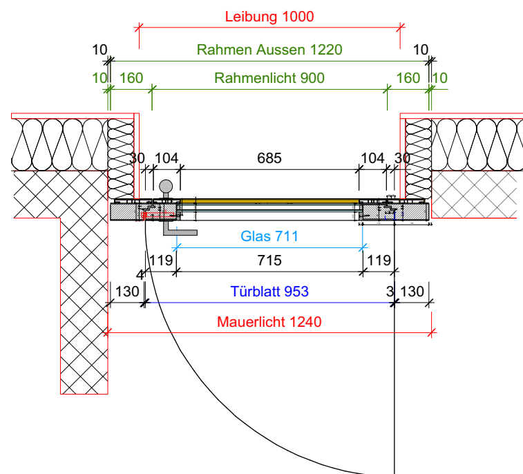
Typ 6-Balkontüre
